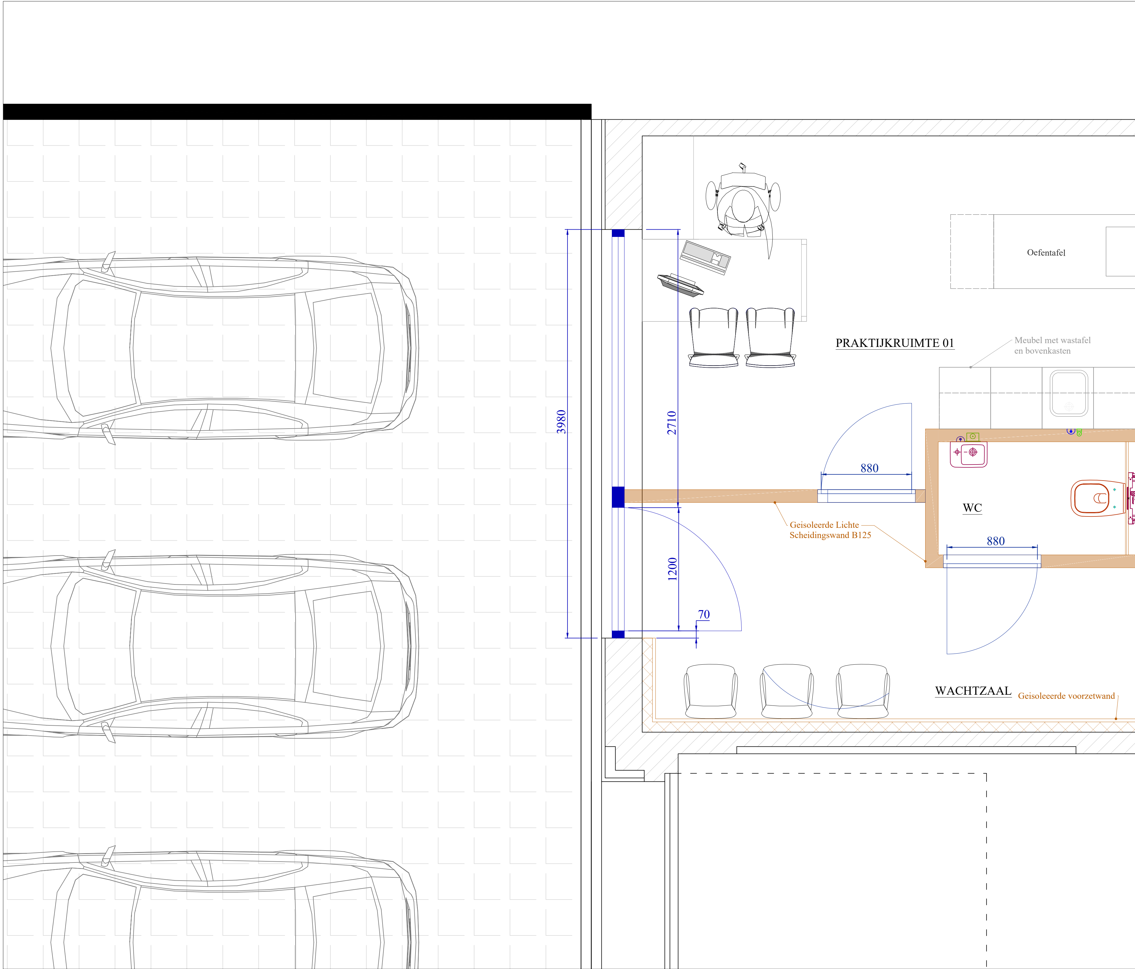
GRONDPLAN GELIJKVLOERS
